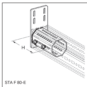
STA F 80-E
